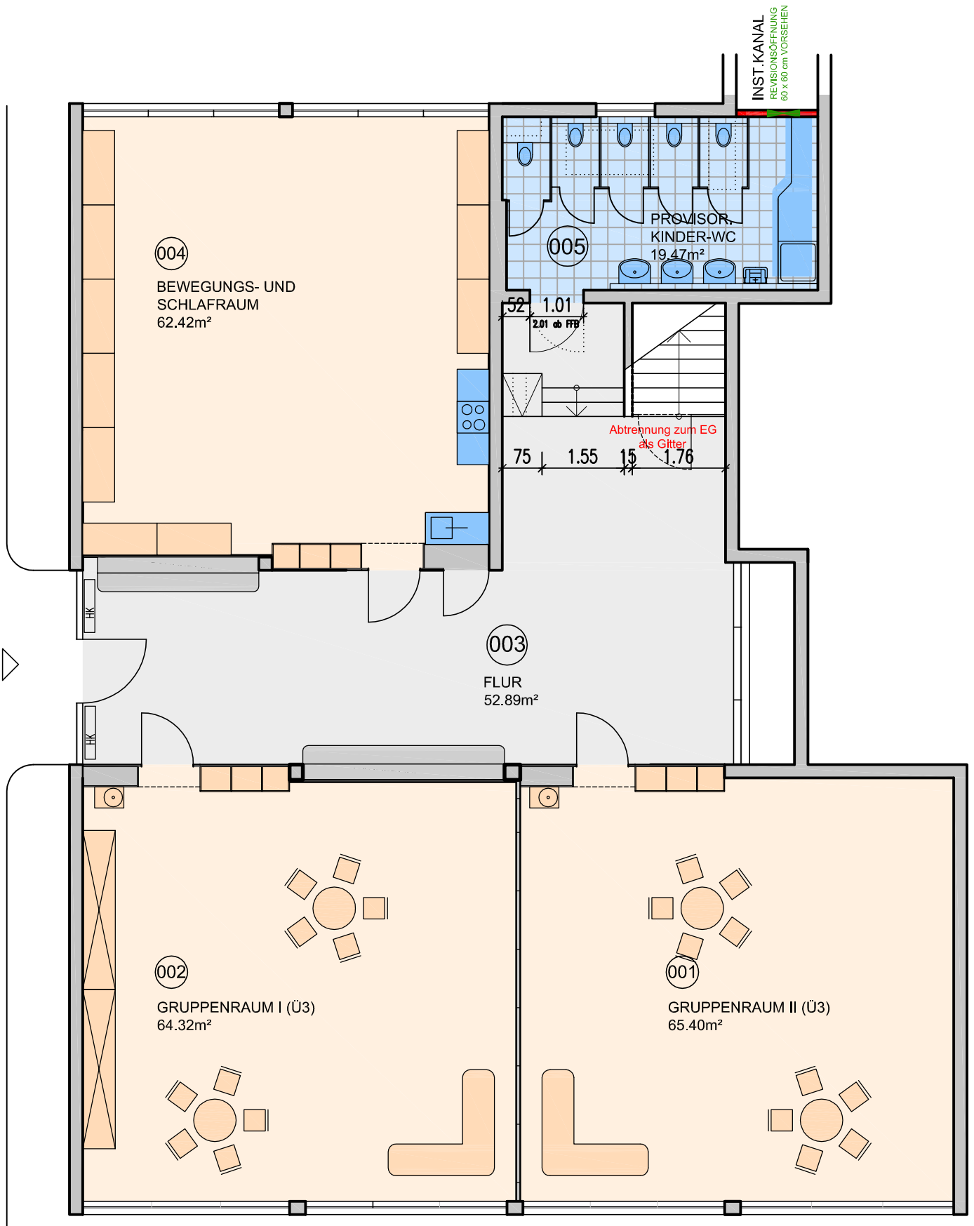
"NEUBAU" GRUNDRISS GARTENGESCHOSS M 1:100
